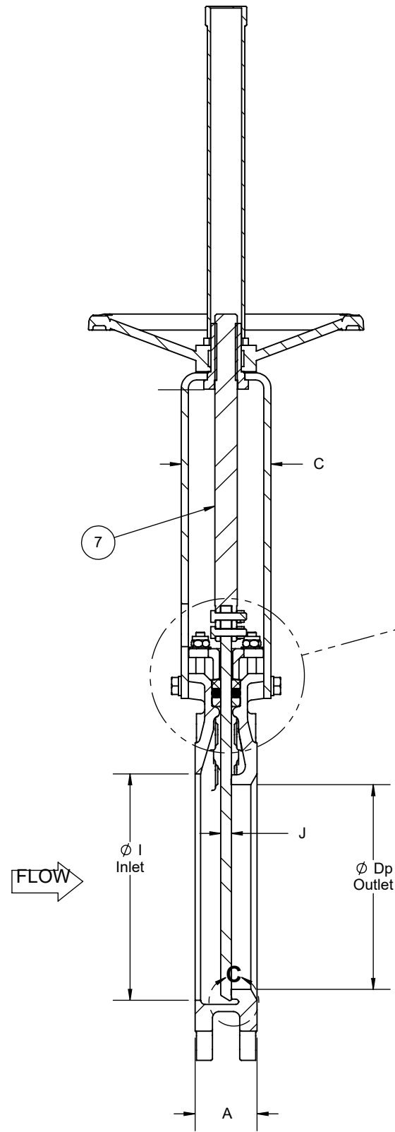
SECTION A-A SCALE 1 : 6
