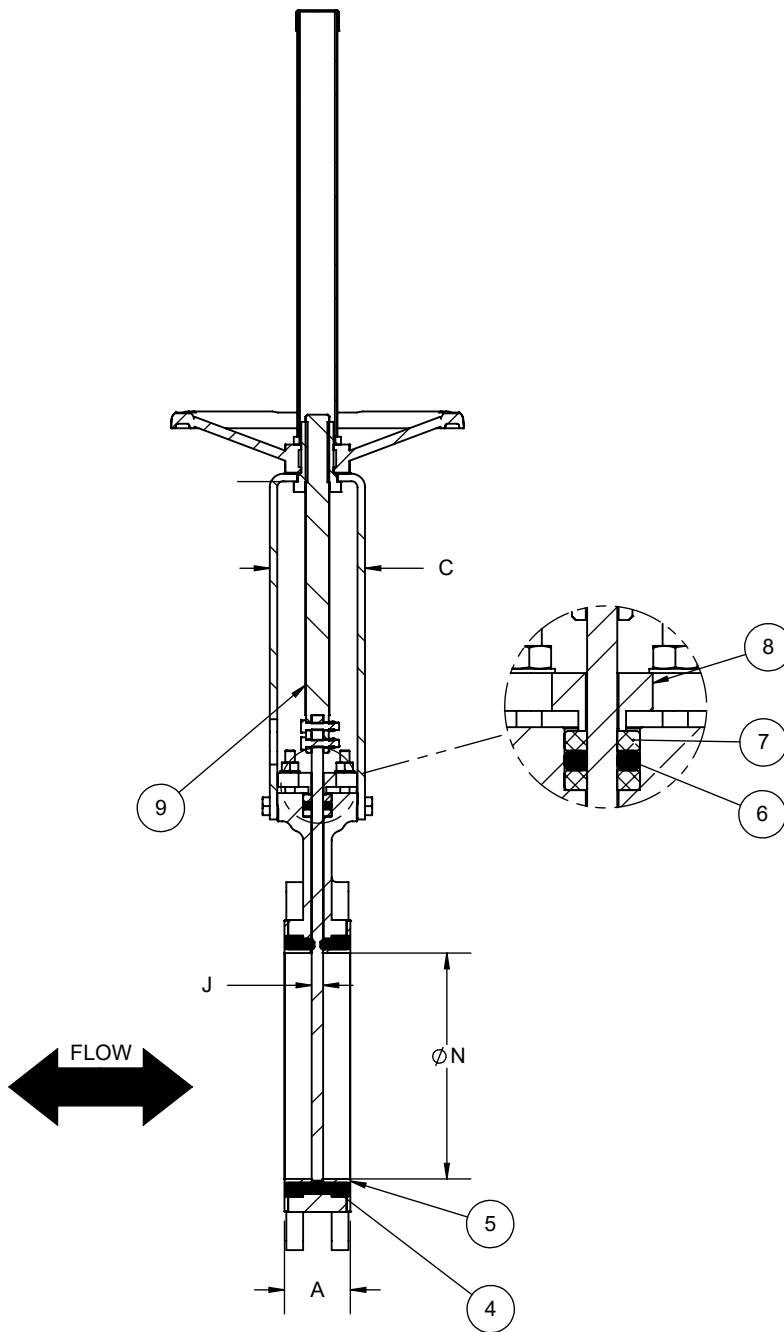
SECTION A-A SCALE 1 : 8
